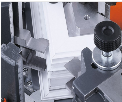
Eckverbindungspresser EP 124
