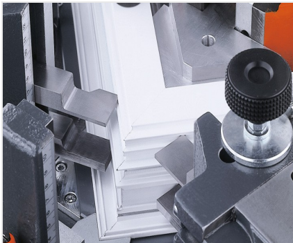
Eckverbindungspressen EP 124
