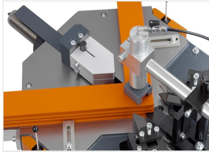
Eckverbindungspressen EP 120
