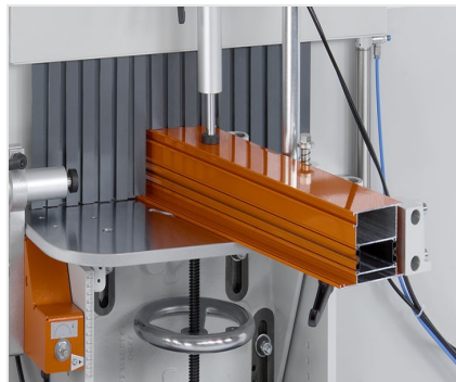
Auslinkfräse AF 223/01
