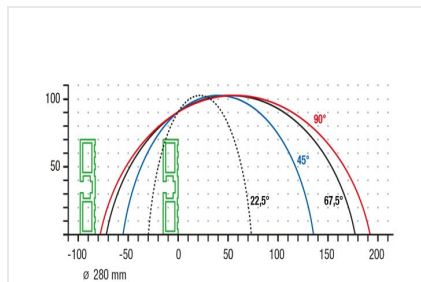
Stolní pila TS 161/21
