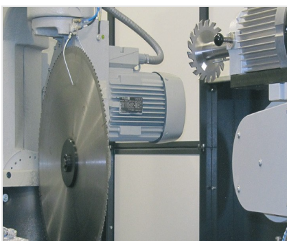
Centrum pro obrábění tyčí SBZ 631
