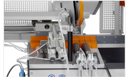
Pilový automat SA 73/36
