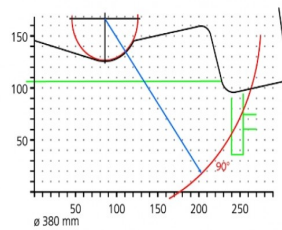
Pilový automat SA 73/36
