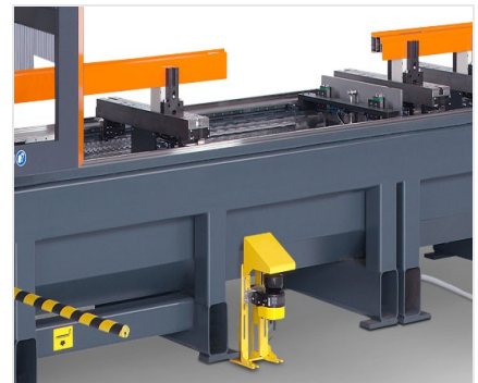
SBZ 140 Centrum pro obrábění tyčí
