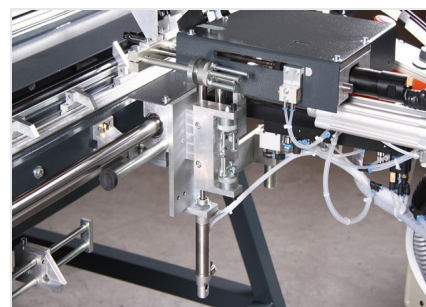
Šroubovací jednotka s nátrubkem s trychtýřem pro ruční vhazování (volitelné příslušenství)
