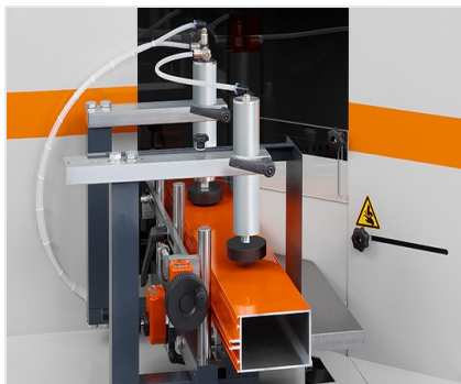
Vyřezávací pila AKS V-550
