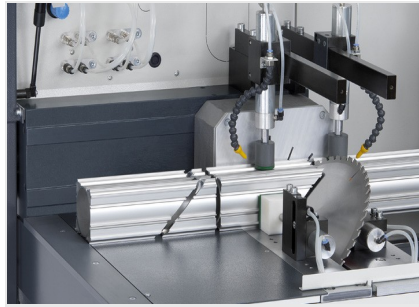
Scie automatique SAS 142/43
