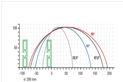
Sierra de mesa TS 161/21
