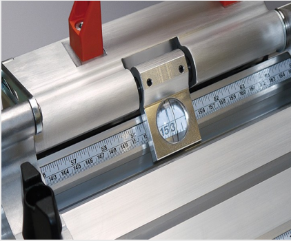
Sistema de tope y medición MMS 100
