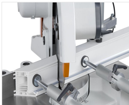
Tronzadora MGS 73/33
