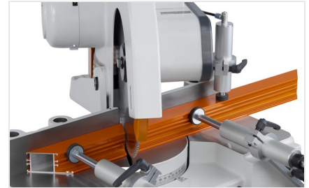
Tronzadora MGS 73/33
