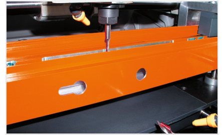
Copiadora fresadora doble KF 78/23
