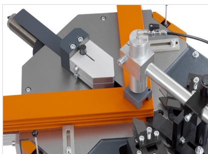
Ensambladora de esquinas EP 120
