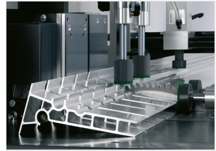
Sägeautomat SAS 142/44
