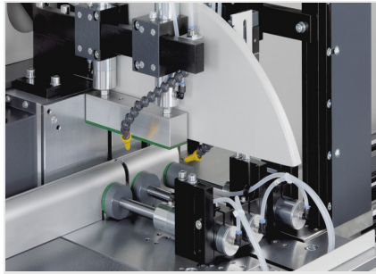
Säageautomat SAS 142/44
