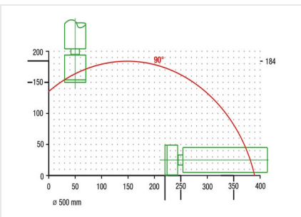
Säageautomat SAS 142/44
