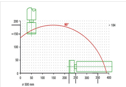
Säageautomat SAS 142/44
