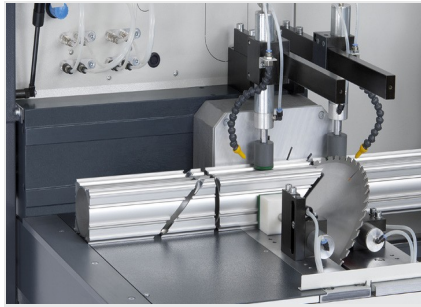
Säageautomat SAS 142/43
