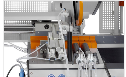
Sägeautomat SA 73/36
