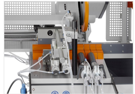
Sägeautomat SA 73/36
