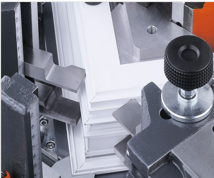
Eckverbindungspresser EP 124
