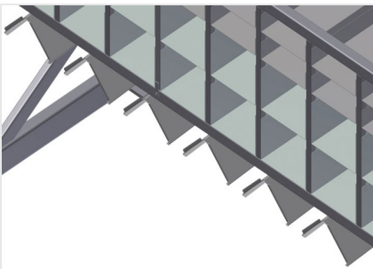
Winkelauflage
