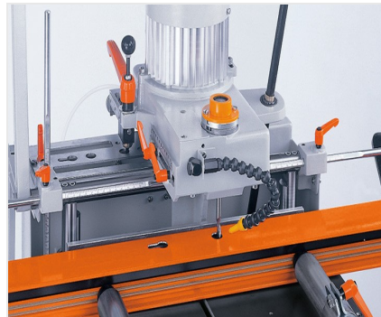
1-Spindel-Kopierfräse AS 70/44
