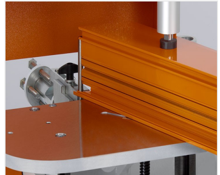
Auslinkfräse AF 223/01
