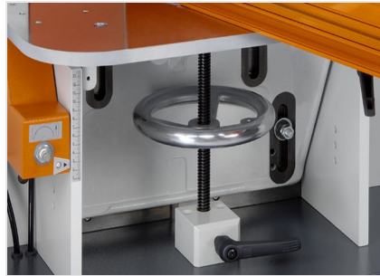
Auslinkfräse AF 223/01
