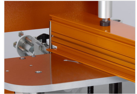
Auslinkfräse AF 223/01
