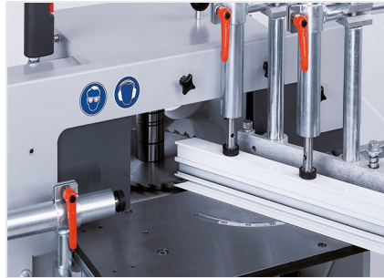
Auslinkfräse AF 222/02
