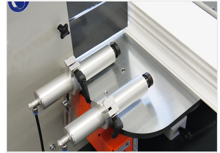
Auslinkfräse AF 222/02
