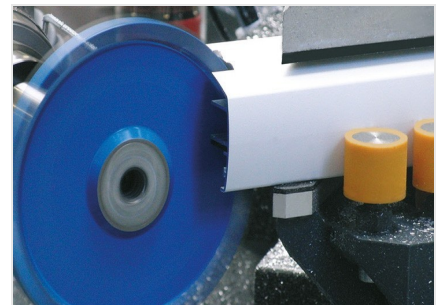
Centrum pro obrábění tyčí SBZ 631
