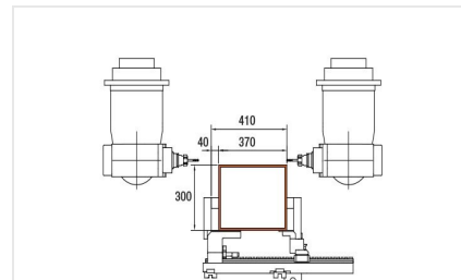
Centrum pro obrábění tyčí SBZ 151 Edition 90
