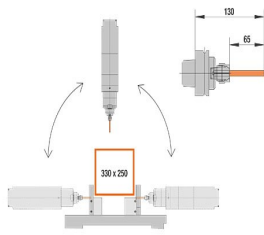
SBZ 140 Centrum pro obrábění tyčí
