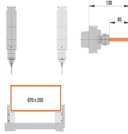
SBZ 140 Centrum pro obrábění tyčí
