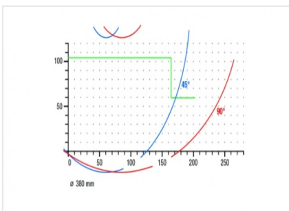
Pokosová pila MGS 73/33
