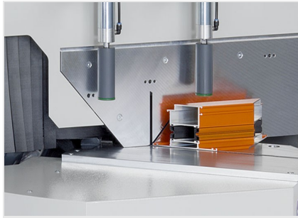
Pokosová pila MGS 105
