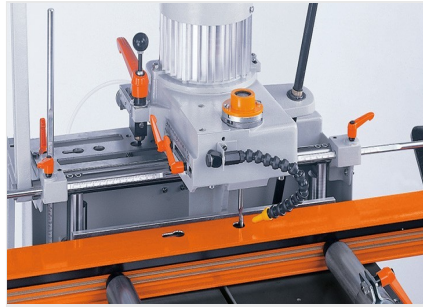
1vřetenová kopírovací fréza AS 70/44
